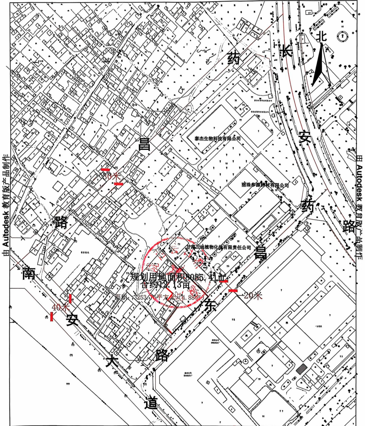
药昌东路西侧、南安大道以北拟出让宗地位置平面图
